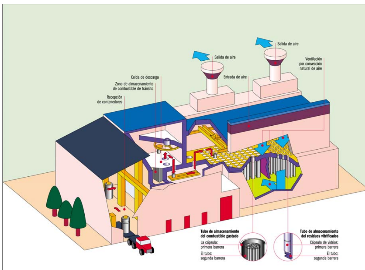
FIGURA 8. ESQUEMA ATC BÓVEDAS
