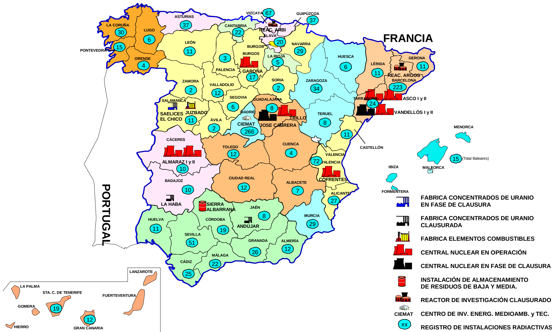
FIGURA B.1. INSTALACIONES GENERADORAS DE RESIDUOS RADIACTIVOS EN
