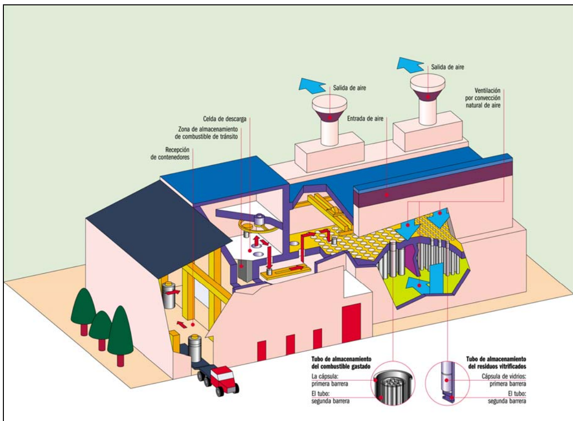
ESQUEMA ATC BÓVEDAS
