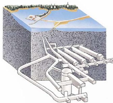
SFR (SUECIA)
