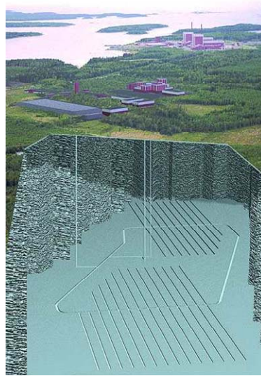
OLKILUOTO (FINLANDIA)
