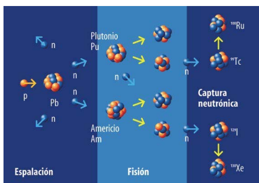
FIGURA 9. SISTEMA DE TRANSMUTACIÓN
